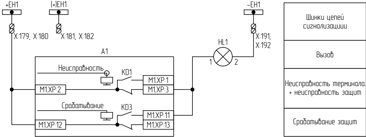
Цепи сигнализации
