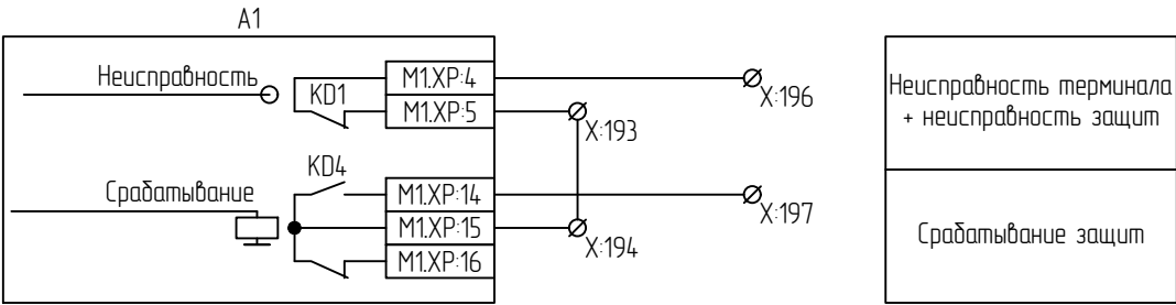
Цепи РАС
