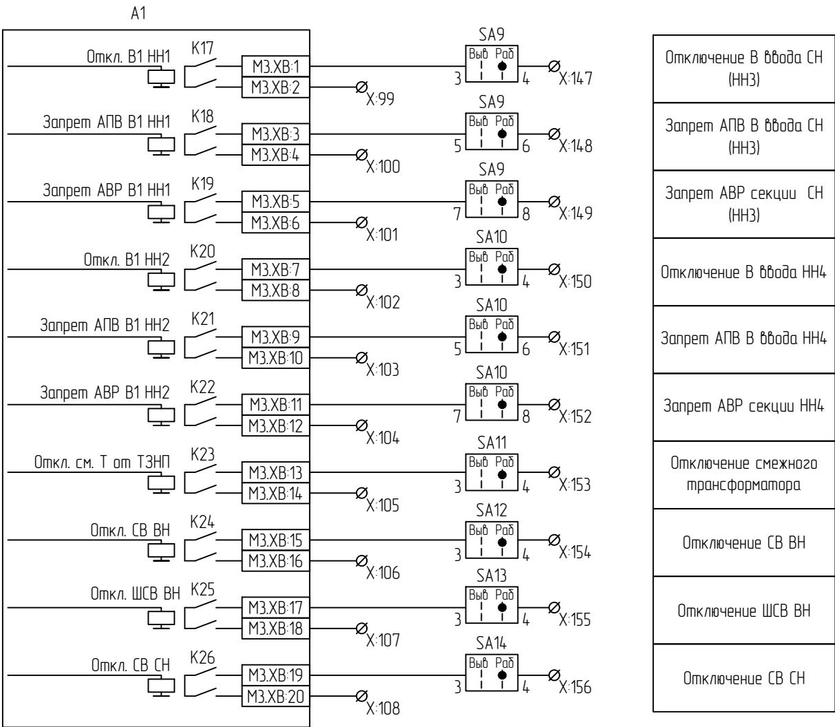
Выходные цепи
